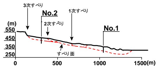
図-3 断面図(現場A)
