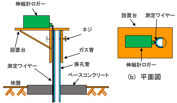
(a) 正面図 図-2 特製設置台(保孔管外周に沿わせたタイプ)の概要
