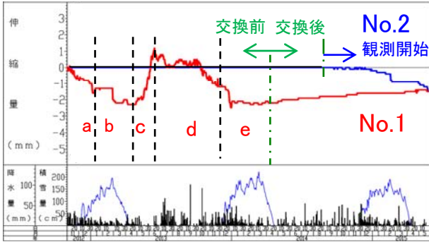
図-4 地中伸縮計変動図(現場 A)
