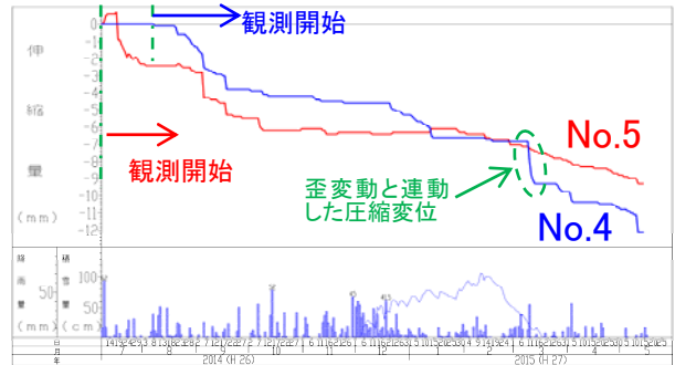
図-8 地中伸縮計変動図(現場 C)
