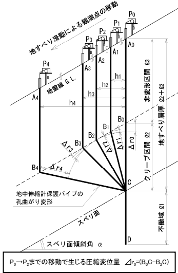
図-1 地中伸縮計観測モデル図 2) に加筆
