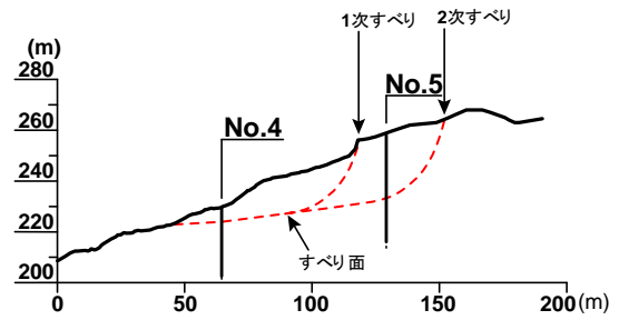
図-7 断面図(現場 C)
