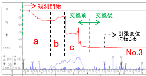
図-6 地中伸縮計変動図(現場 B)
