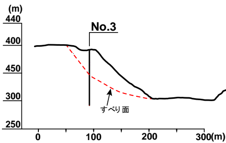
図-5 断面図(現場 B)
